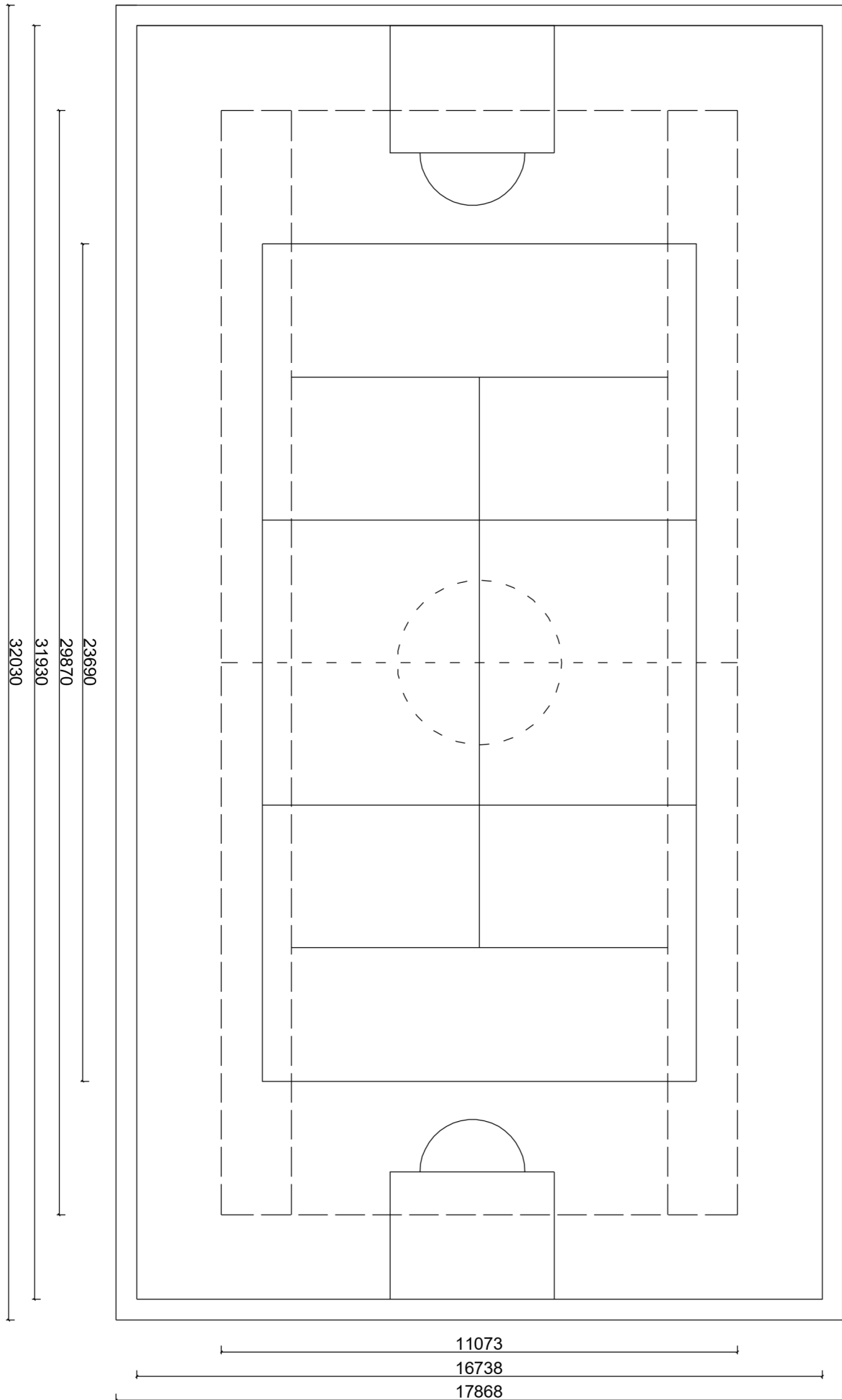
Plan sytuacyjny boiska wielofunkcyjnego
